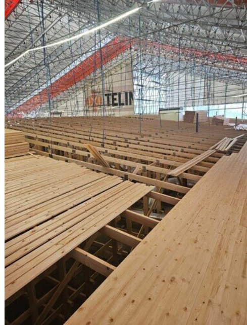
Vielä riittää raakapontin asennusta
