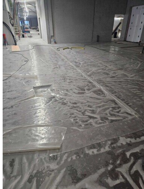
Maanvaraiset laatat valettu, tähän tulee kiilloitettu betonilattia
