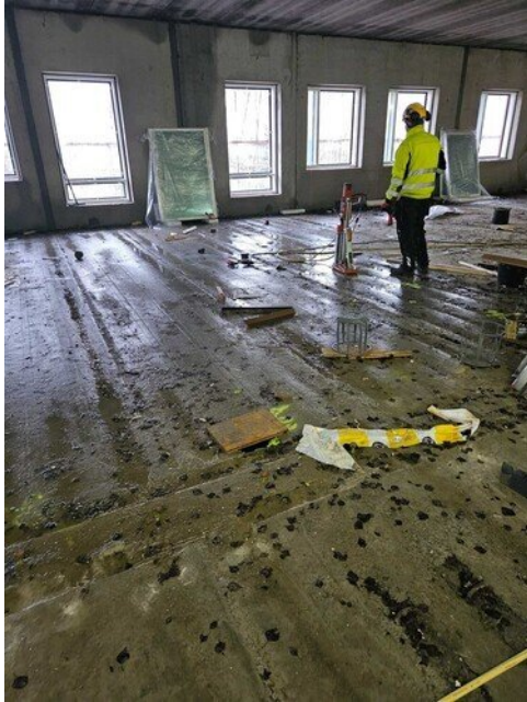
Timanttikorari työssä, 2 kerroksen lattiaan viemäreille reikiä
