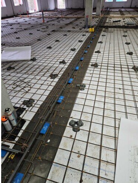
Liikuntasaumaraudoitteet asennettuna
