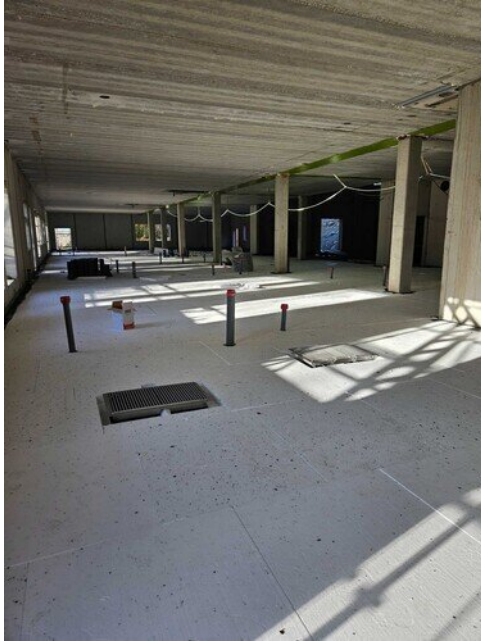
Lattiaeristettä asennettu
