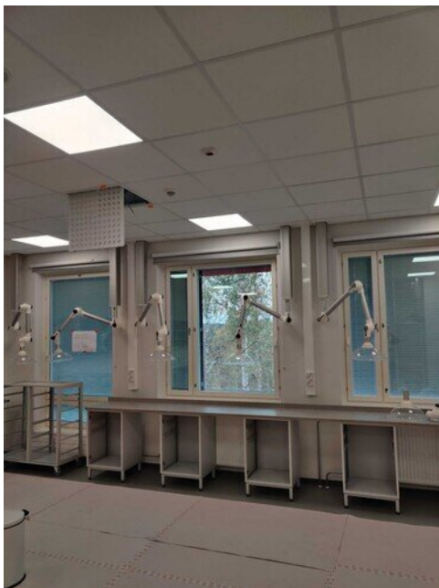
Kohdepoistojen asennus
