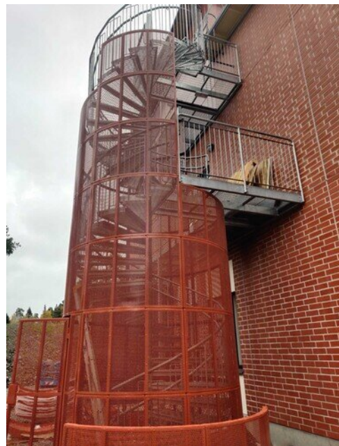
Kierreportaiden ulkokehikon asennus käynnissä
