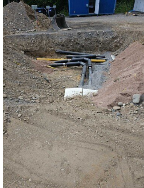
Kaukolämpöliitokset koeponnistettu, eristys puuttuu
