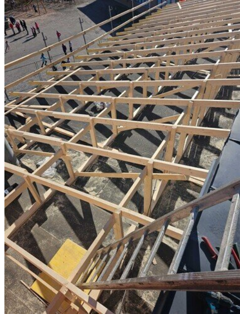
Vanhan osan tasakatonle tehdään pulpettikatto
