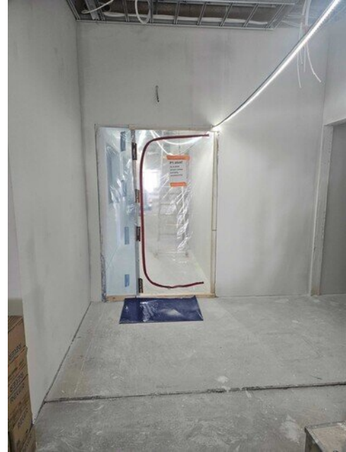
2. kerroksessa IV-kanava-asennukset pölypuhtaassa tilassa muovi-oven takana
