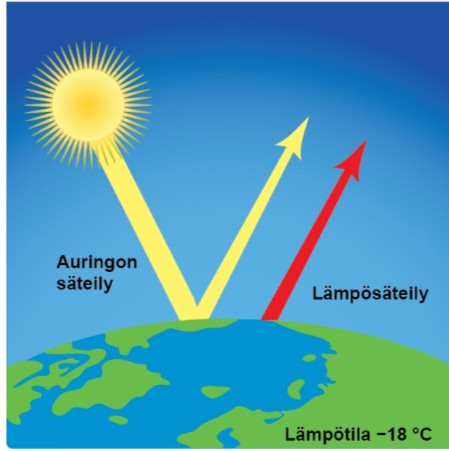
Ilman kasvihuoneilmiötä
