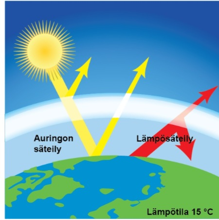
Kasvihuoneilmiön kanssa
