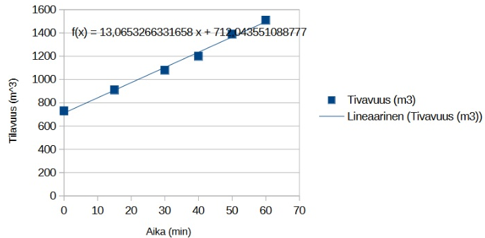
Siilon tilavuus ajan funktiona
