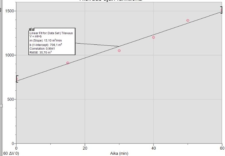
Tilavuus ajan funktiona
