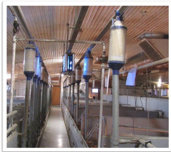
Sikalan ruokintajärjestelmä
