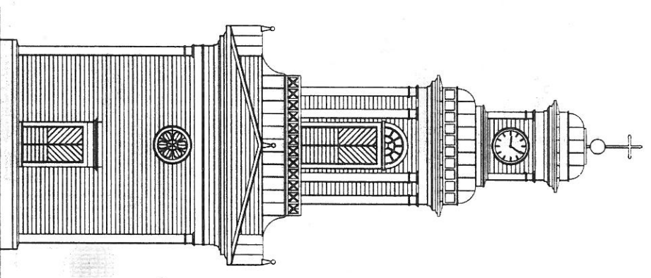
JULKISIVU ETELÄÄN
