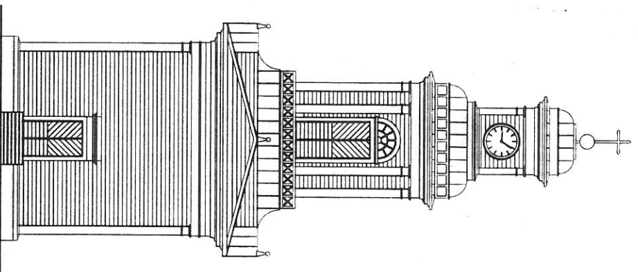
JULKISIVU POHJOISEEN
