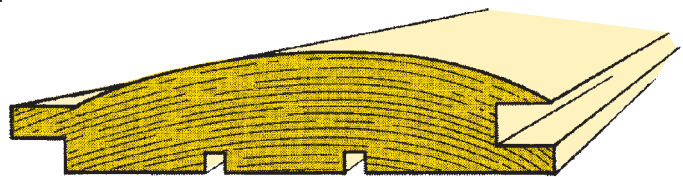
hirsipaneeli
