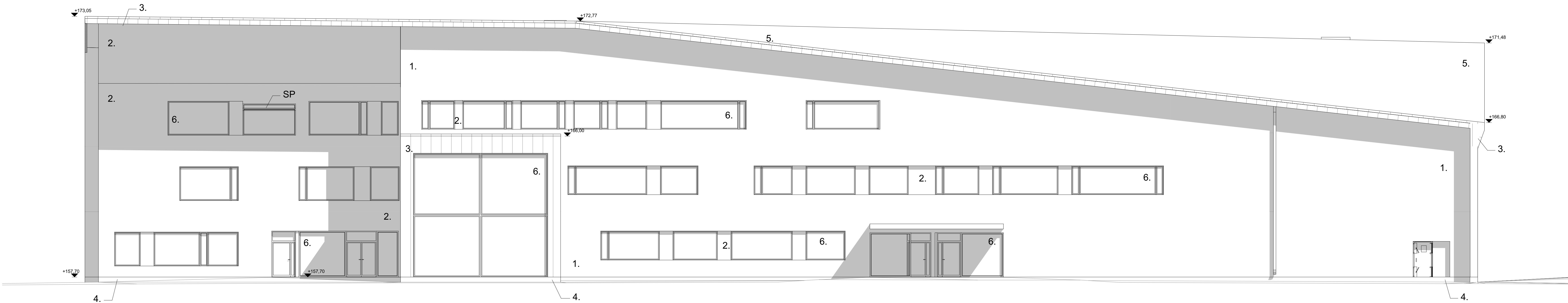
JULKISIVU ITÄÄN 1:100
