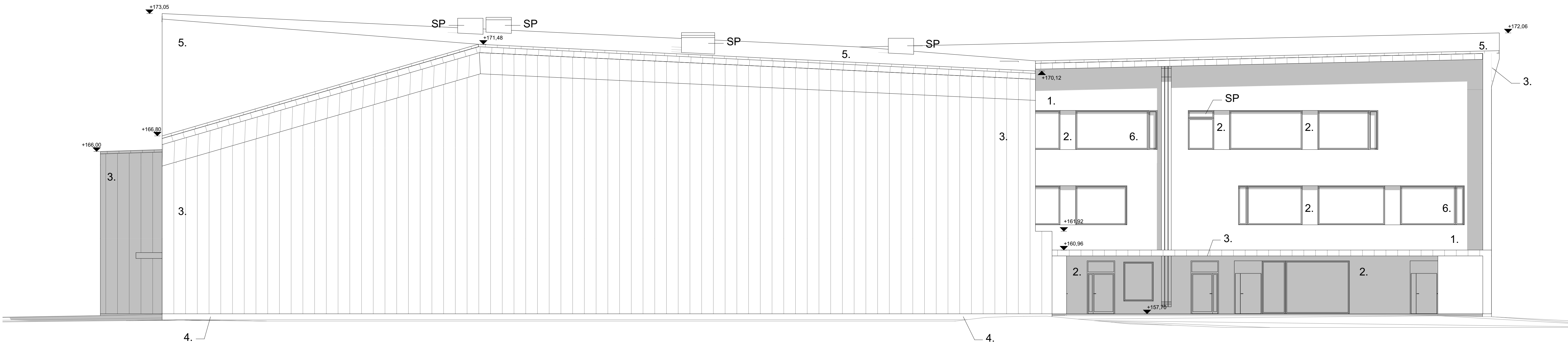
JULKISIVU POHJOISEEN 1:100
