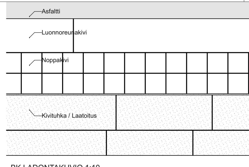
BK LADONTAKUVIO 1:10
