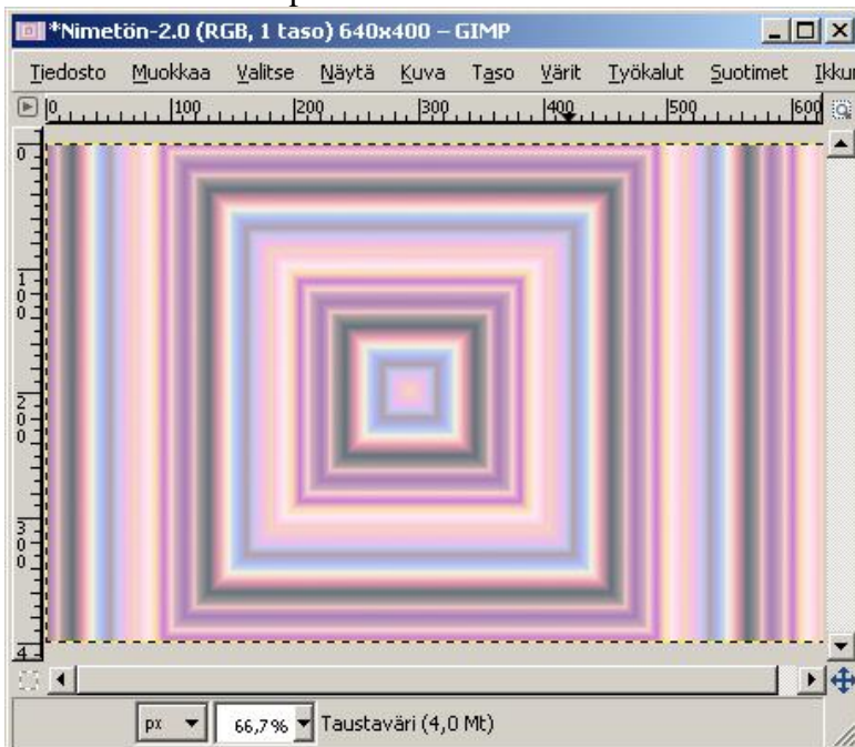
Kuva 4. Neliökuviot pastelliväreillä
