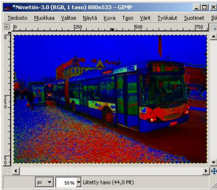
Kuva 7. Max RGB-toiminto
