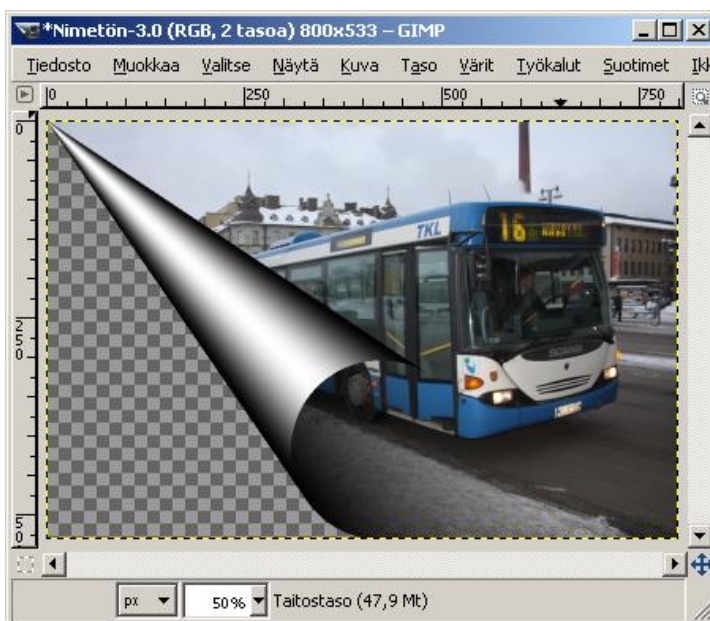
Kuva 6. Koirankorva
