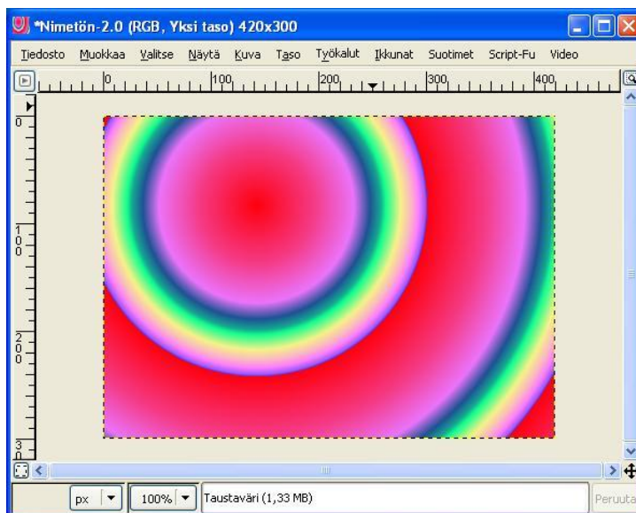
Kuva 1. Pallomainen väriliukuma
