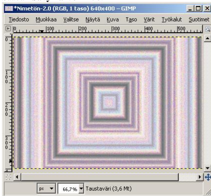
Kuva 5. Värimuunnoksia: HSV-kohina.
