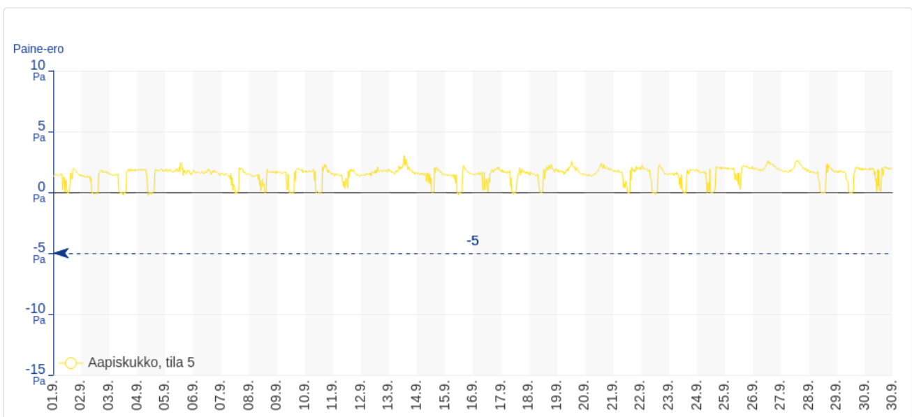
Paine-ero ulkovaipan yli, Aapiskukko, syyskuu 2020.
