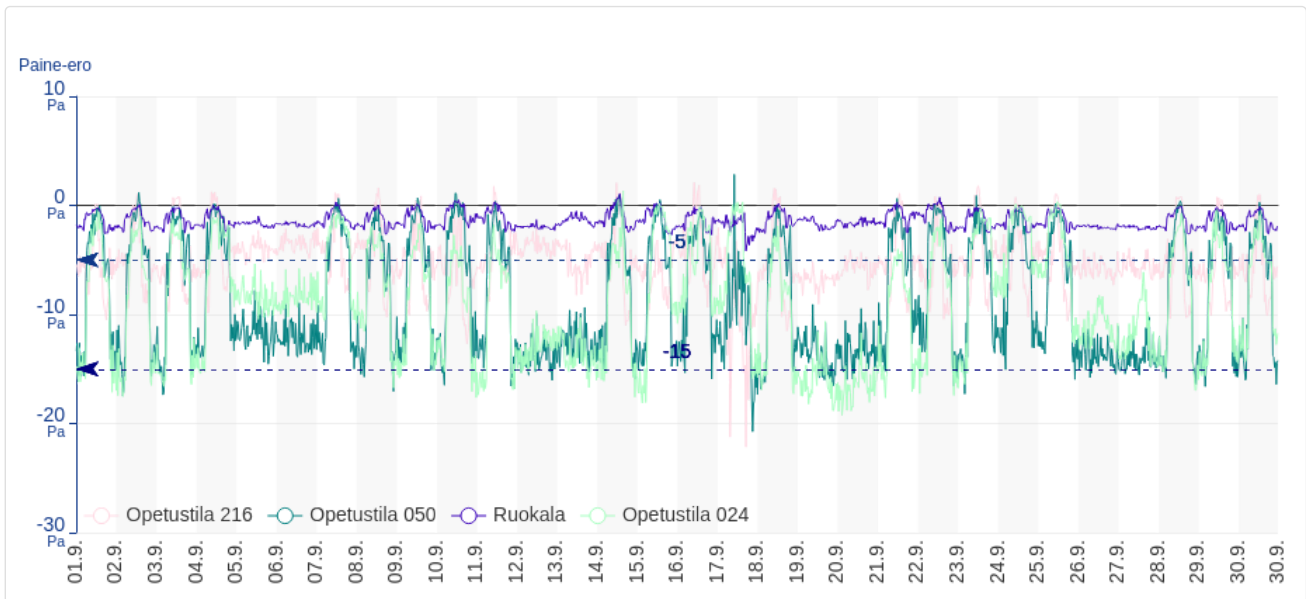
Paine-ero ulkovaipan yli, vanha puoli, syyskuu 2020.
