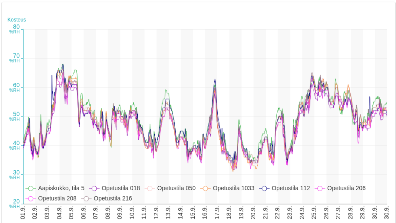
Suhteellinen kosteus, syyskuu 2020.
