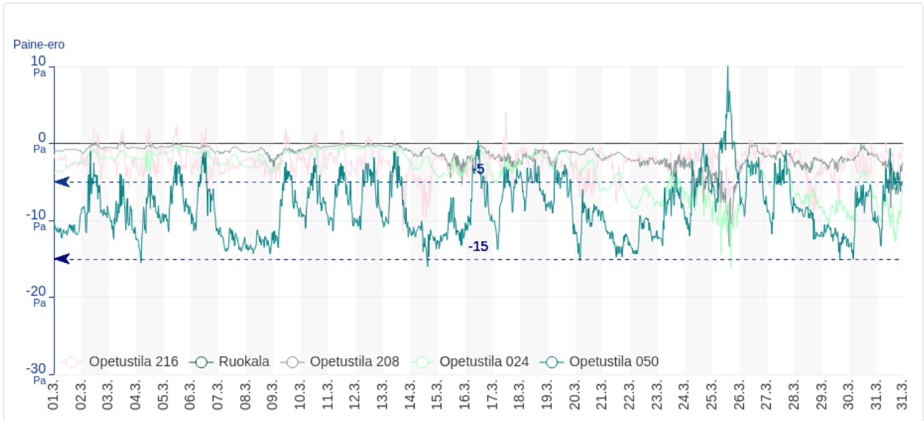
Paine-ero ulkovaipan yli, vanha puoli, maaliskuu 2020.
