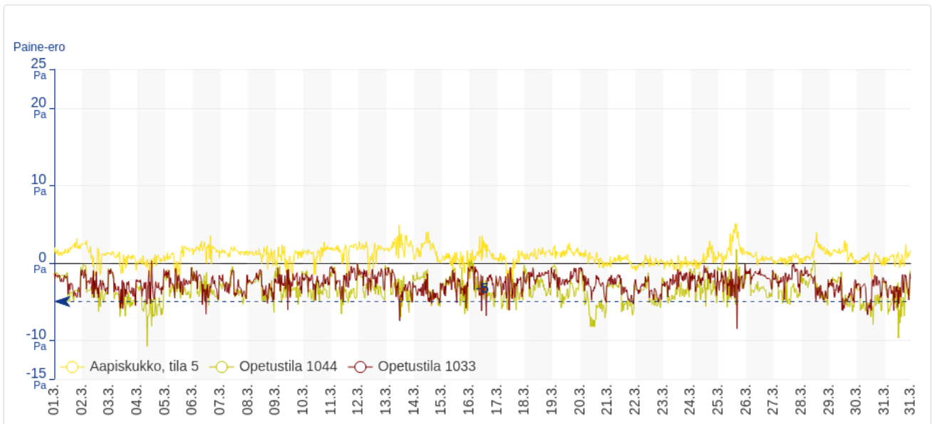
Paine-ero ulkovaipan yli, uusi puoli ja Aapiskukko, maaliskuu 2020.
