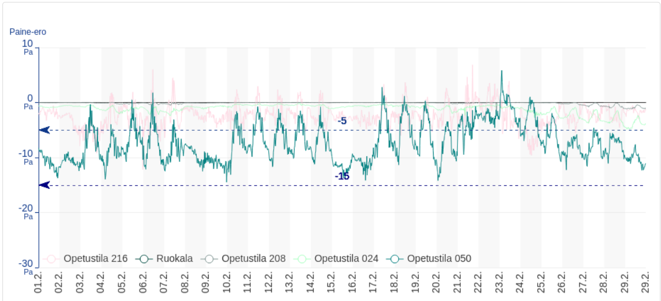
Paine-ero ulkovaipan yli, vanha puoli, helmikuu 2020.
