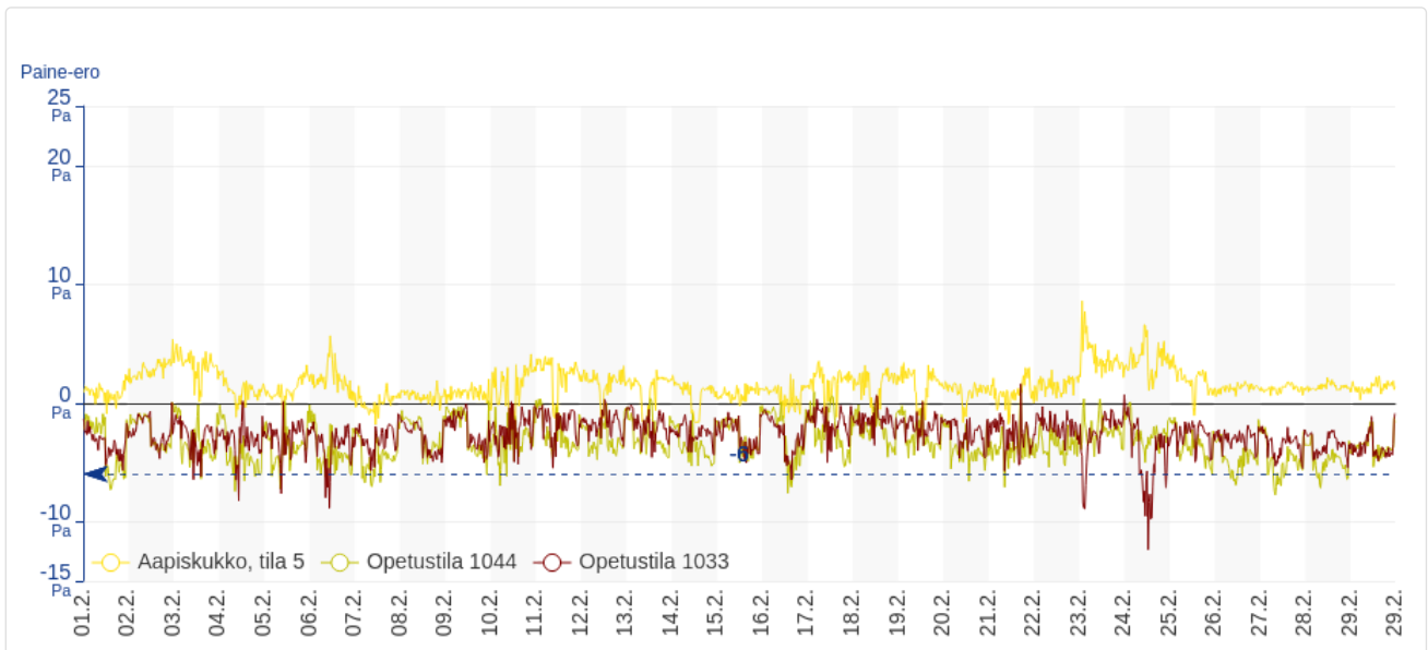
Paine-ero ulkovaipan yli, uusi puoli ja Aapiskukko, helmikuu 2020.
