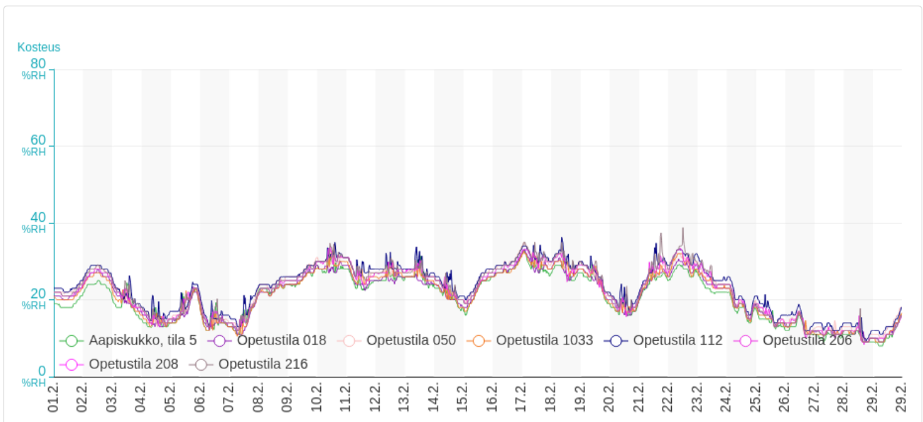
Suhteellinen kosteus, helmikuu 2020.
