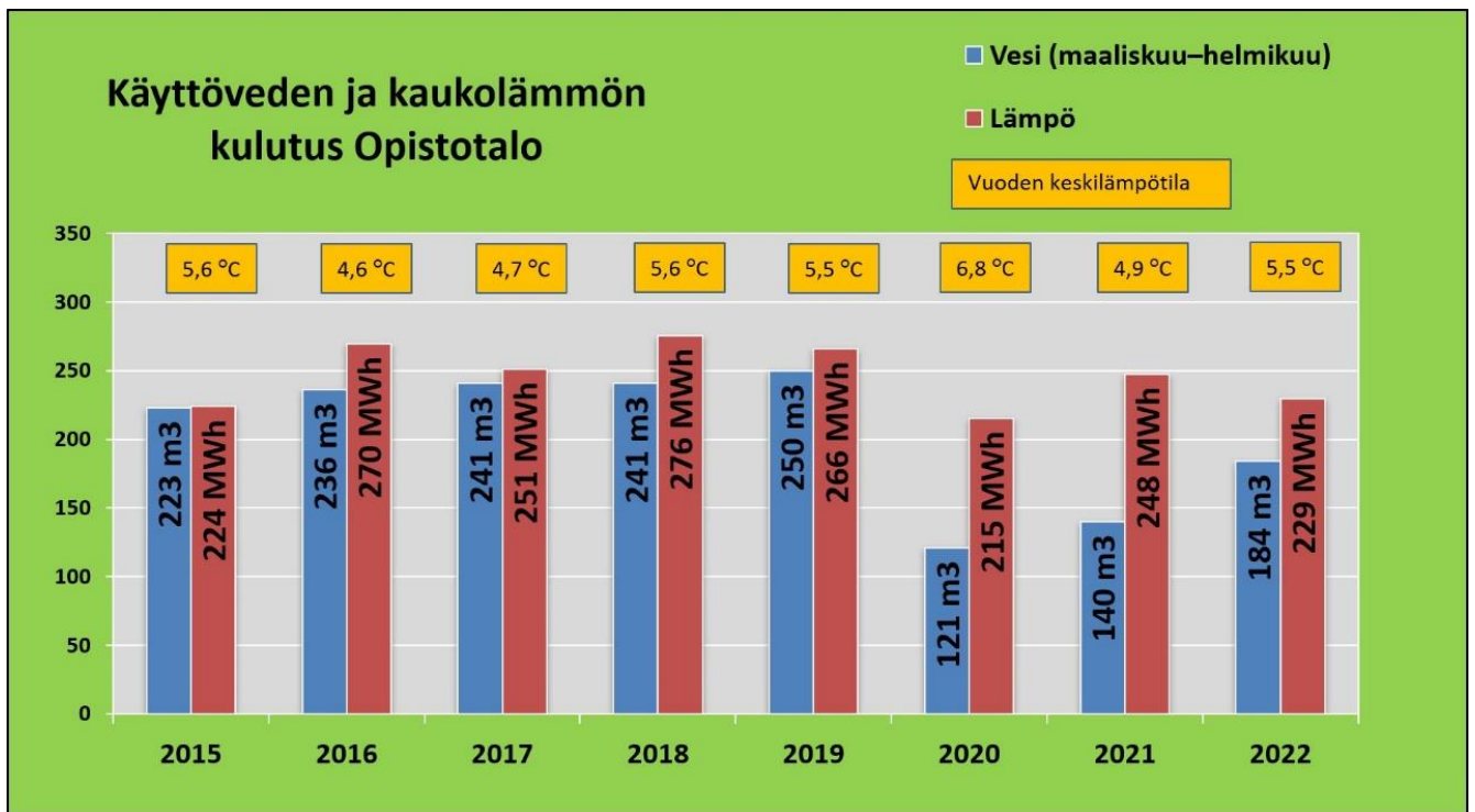
Kuvio 3. Käyttöveden ja kaukolämmön kehitys EKKOssa vuosina 2015–2022
