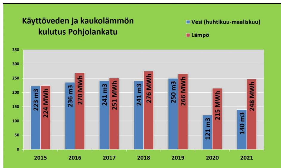
Kuvio 3. Käyttöveden ja kaukolämmön kehitys EKKOssa vuosina 2015–2021
