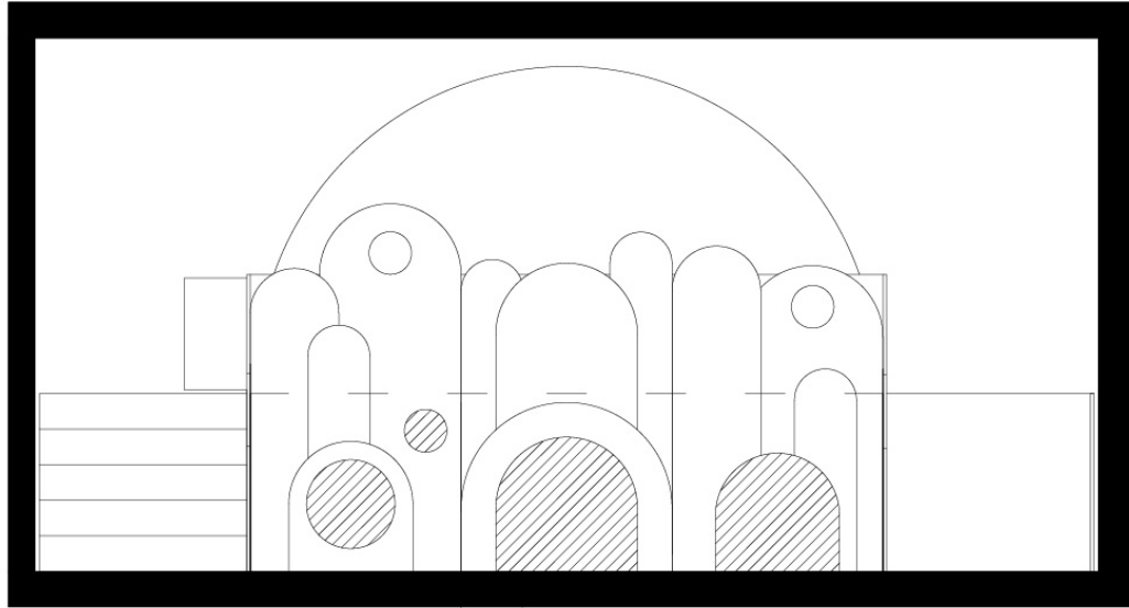
Leikkaus B-B
